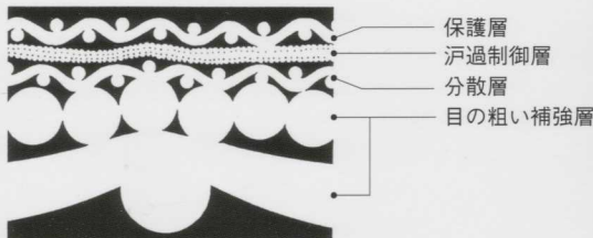
5層積層の断面構造
